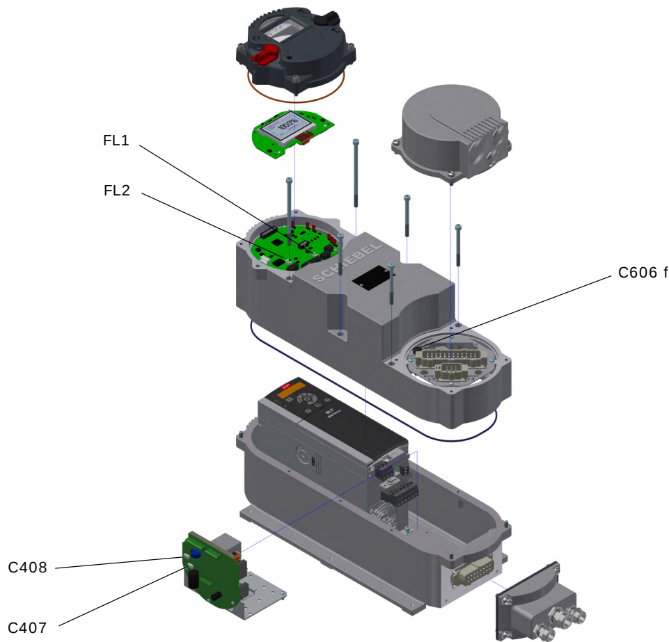
Bild 4: Sicherungen Standardversion
