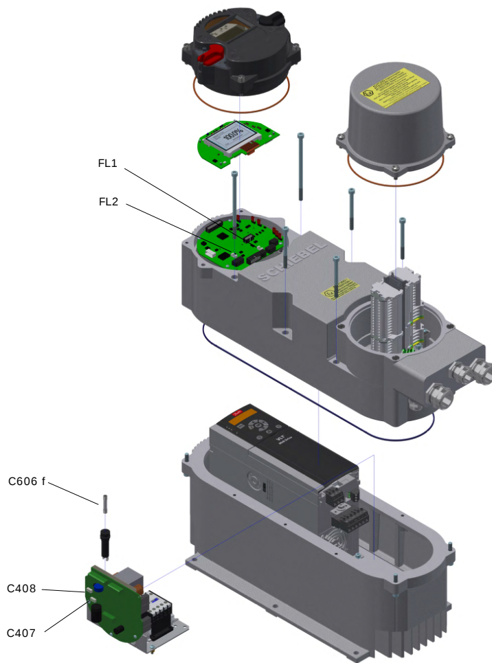
Bild 5: Sicherungen Ex-Version
