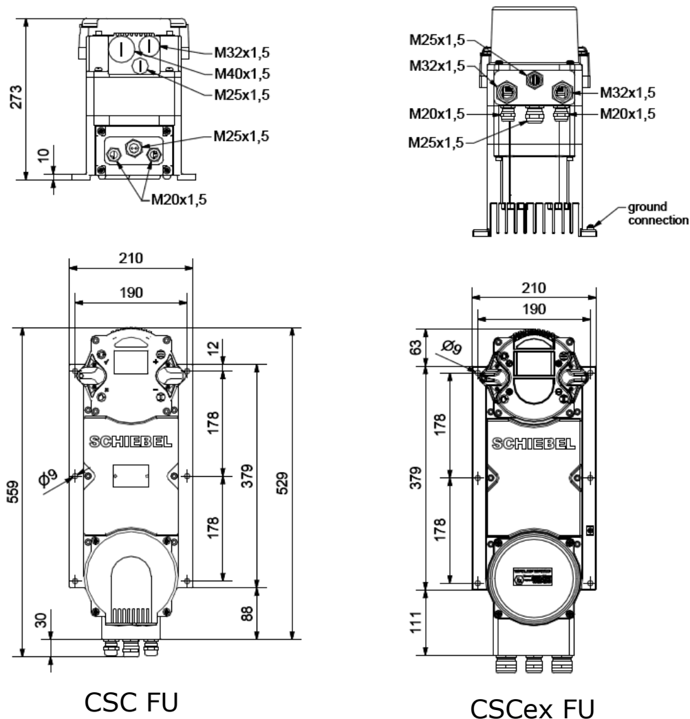
Bild 1: Abmessungen
