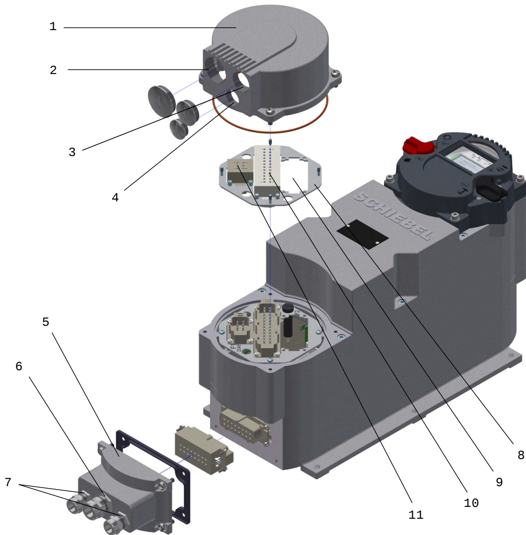
Bild 2: Anschluss Standardversion
